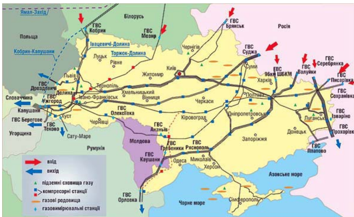
Рис. Схема ГТС України Джерело: newzz.in.ua
